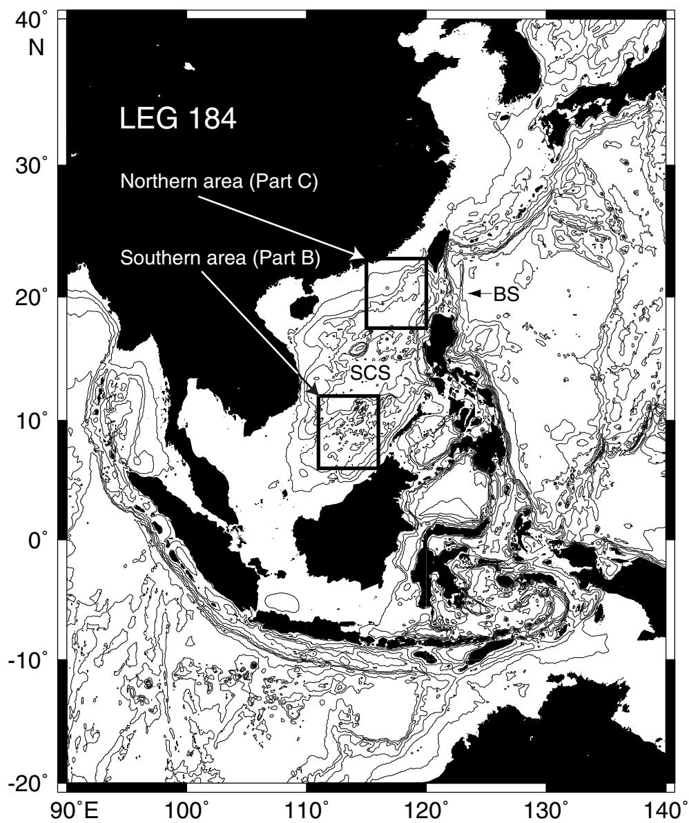
ODP Leg 184 Site Map (Part A) Sites 1143–1148
