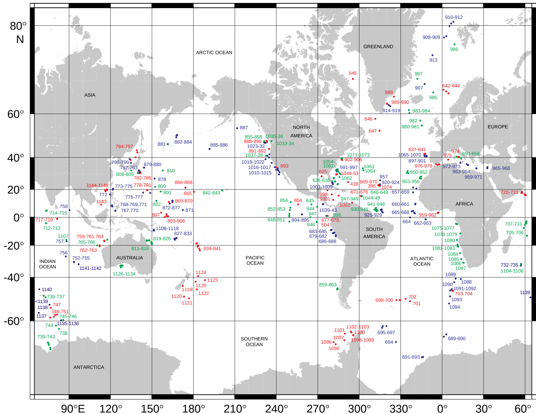
ODP Legs 100-184, Sites 625-1148
